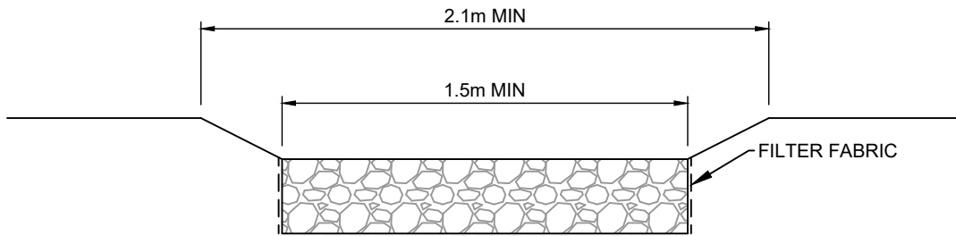
ELEVATION B
