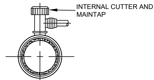
ELECTROFUSION TAPPING SADDLE PE PIPE
